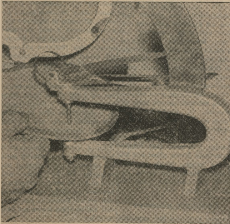
Med det här mätverktyget — som är hemmagjort — mäts stockleken på botten och lock i fiolen. Det är mycket viktigt att mätten är de riktiga.
